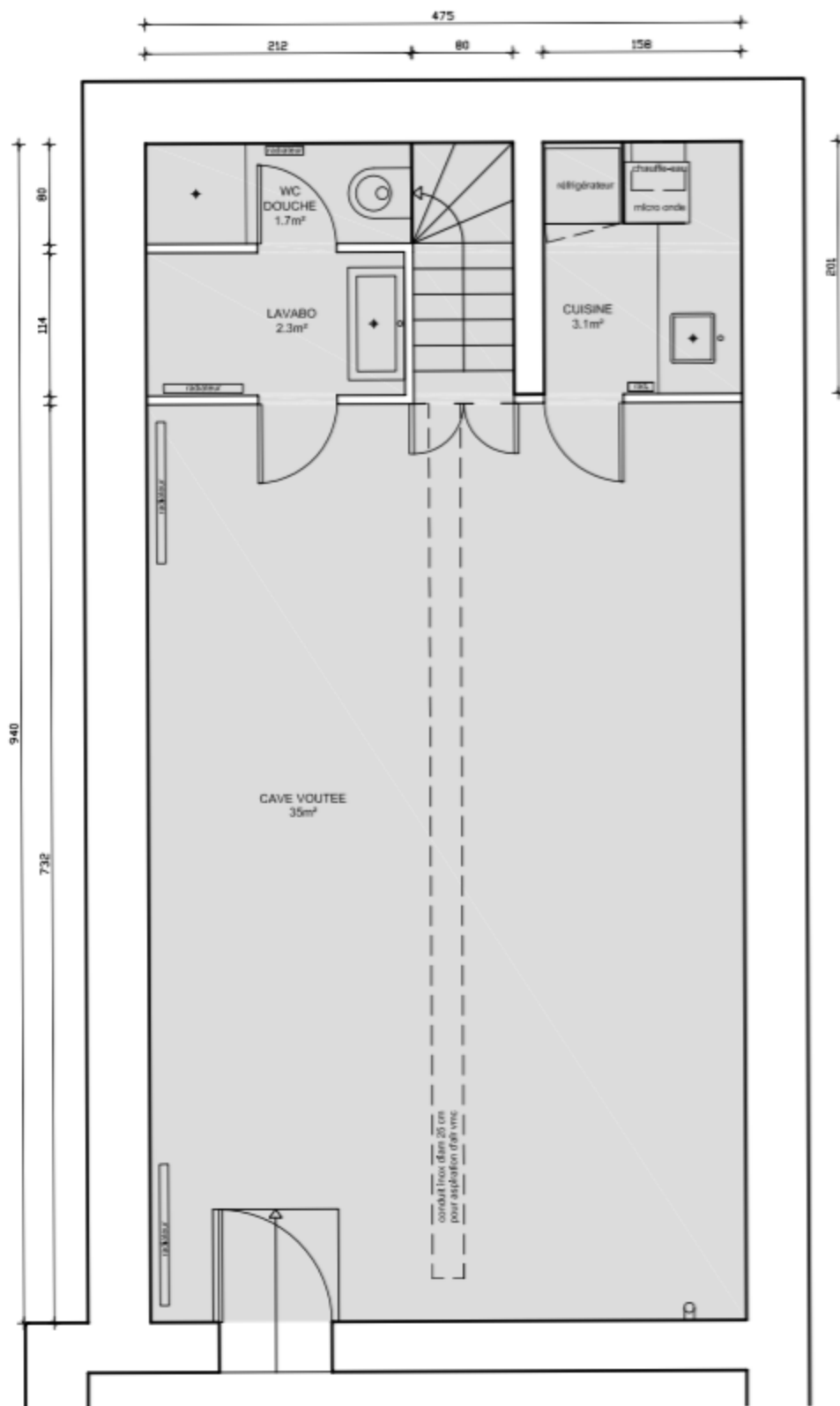
PLAN CAVE VOUTEE, SOUS-SOL
